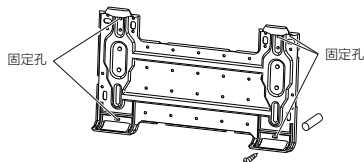
安装板固定螺丝左边两颗，右边三颗，总数不少于五颗。
