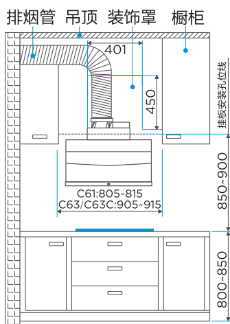
排烟管走橱柜安装示意图
