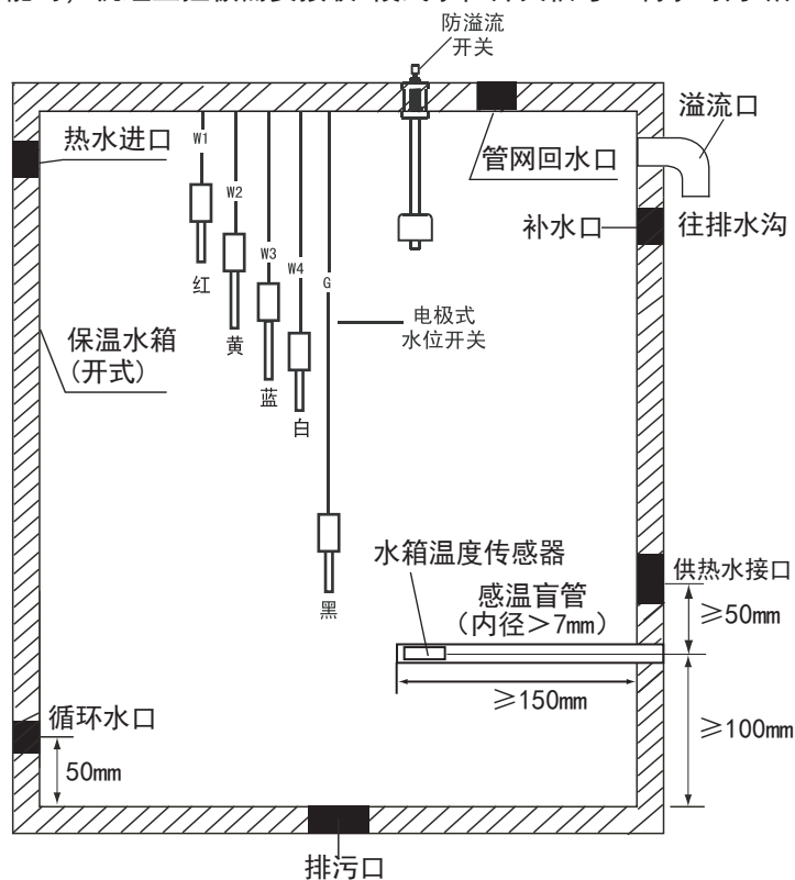
图4.1 水箱简图
