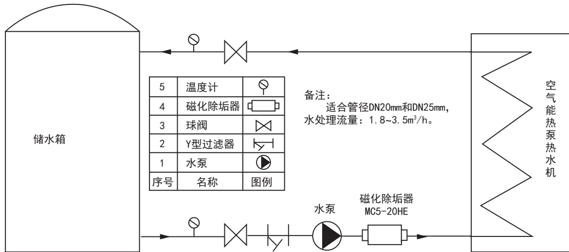
图9.1 磁化器安装示意图 (磁化器建议安装在机组循环进水口)
