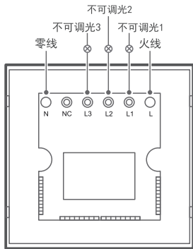
接线示意图
