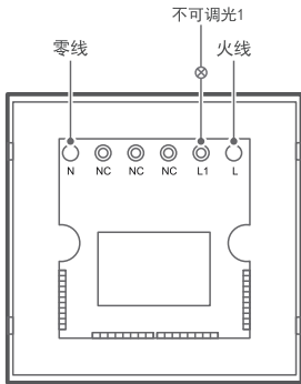
接线示意图
