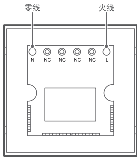
接线示意图
