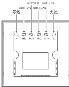
接线示意图
