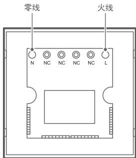
接线示意图
