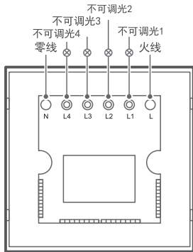
接线示意图
