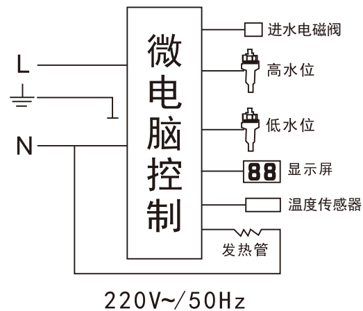
商用电热开水机电路图
