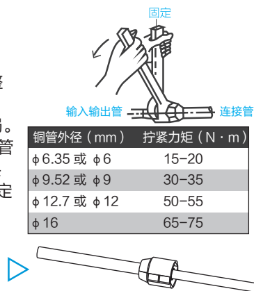
用防拆帽锁紧接头
