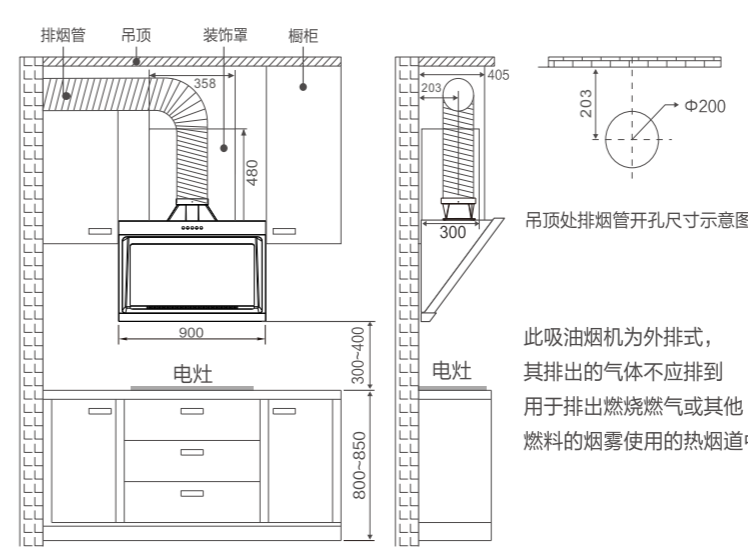
排烟管走橱柜安装示意图
