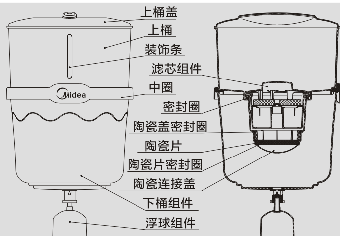
MT-3(865CB)零部件名称
