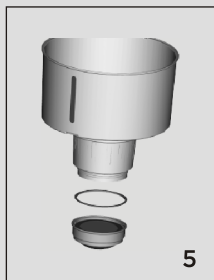
将陶瓷滤芯组件安装在上桶底部（注意请勿丢失陶瓷盖密封圈）
