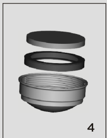
安装陶瓷滤芯组件
