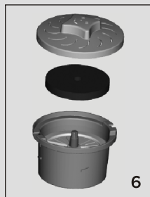
将活性炭纤维片放在专用料滤材盒内，然后箭头相对，扣上滤芯盒盖。转动滤芯盒盖至停止状态，即装好。
