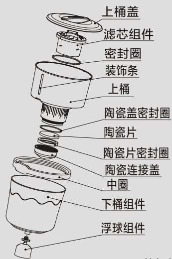
MT-3(865CB)整机爆炸图
