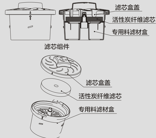
滤芯组件爆炸图
