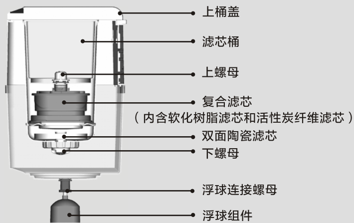
MT-3(870CB)/MT-3(870CB)红色经典 零部件名称
