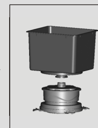
将复合滤芯旋入滤芯桶底部
