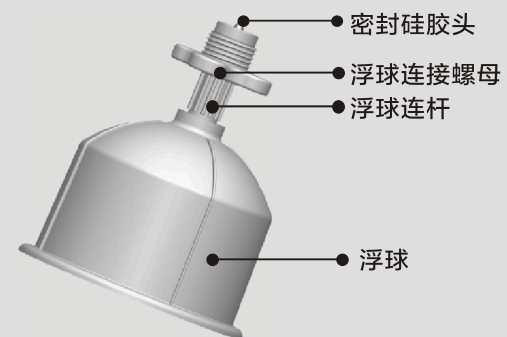
浮球组件图
