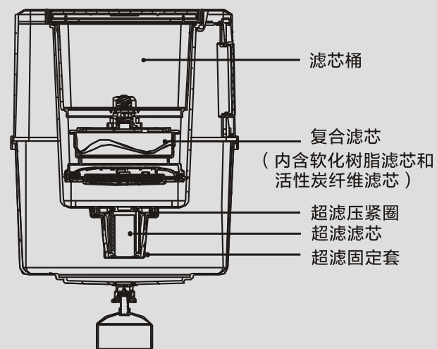
MU-3(875CB)/MU-3(1275CB)零部件名称
