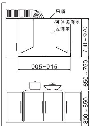
安装方式二：排烟管走吊顶安装示意图
