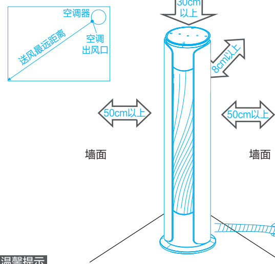
房间空调器使用示意图
