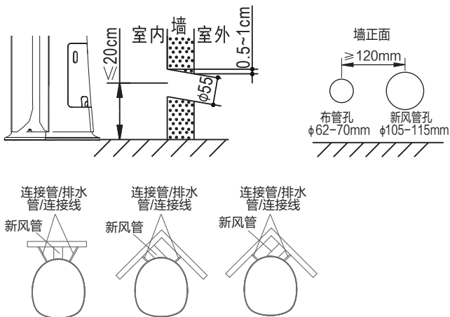
俯视图（图中连接管/排水管/连接线分别表明了左出管及右出管两种形式）
