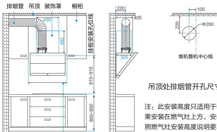
排烟管走橱柜安装示意图
