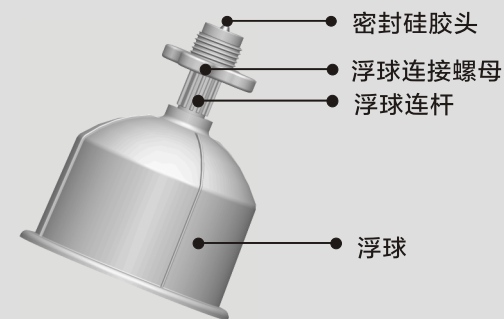
浮球组件图
